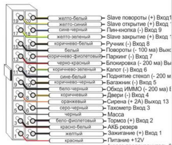
Разъем X7 (Питание / Входы / Выходы)
