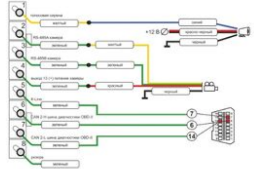
Разъем X 8 вид со стороны проводов
