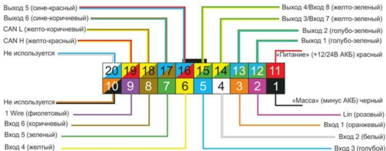
Вид со стороны проводов
