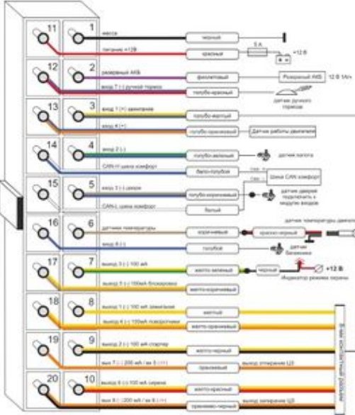
Разъем X 20 вид со стороны проводов
