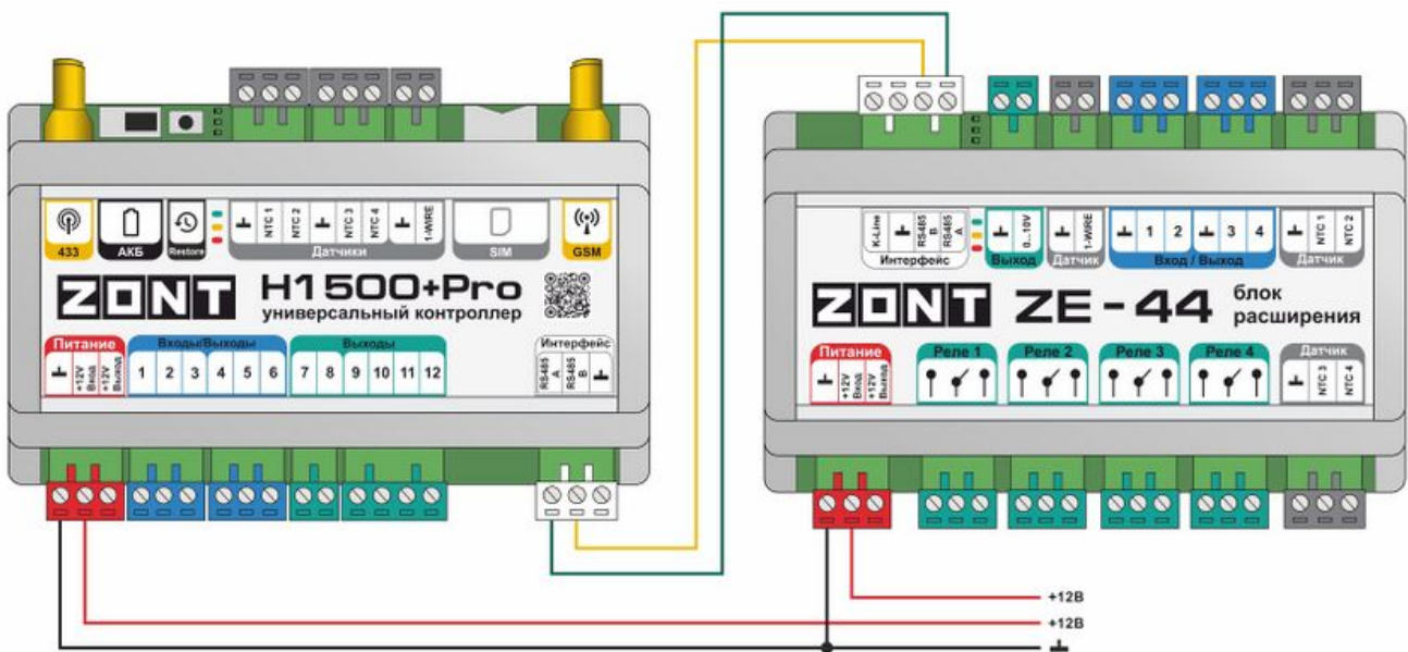
Схема подключения БР и ZONT H1500+PRO по RS-485:
